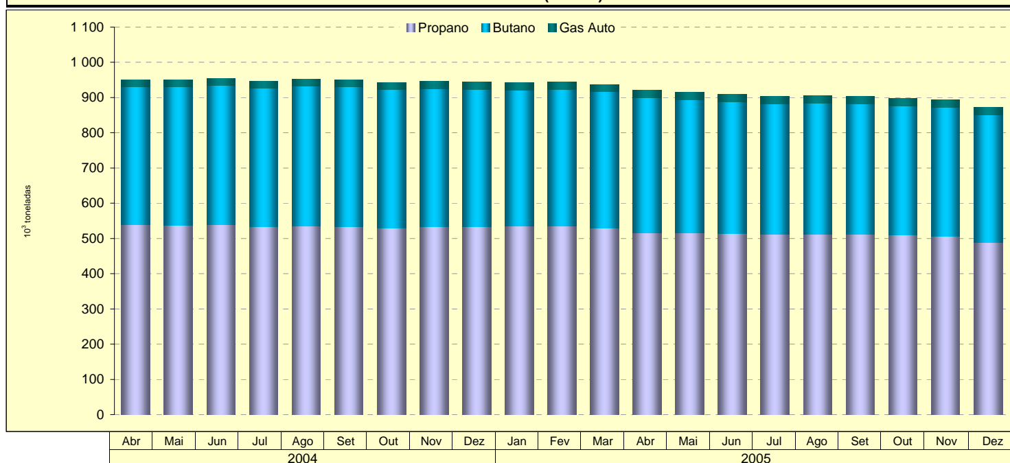
Ano Móvel - GPL (10 3 ton)
