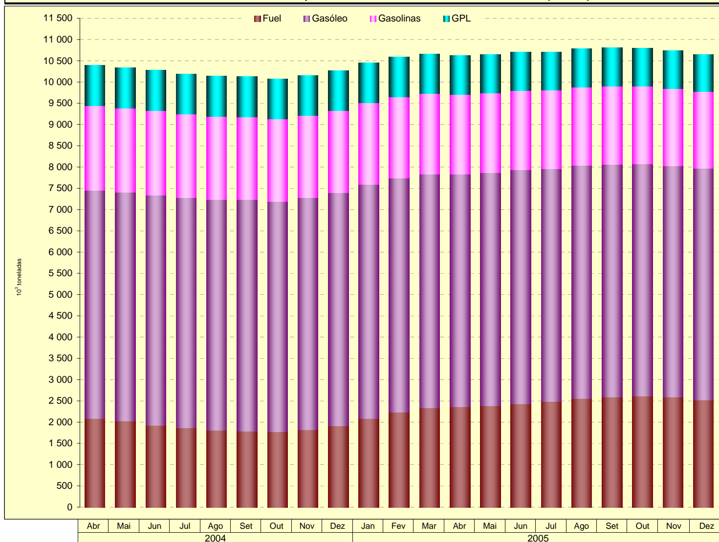
Ano Móvel - Consumo dos Principais Derivados do Petróleo no Mercado Interno (10 3 ton)
