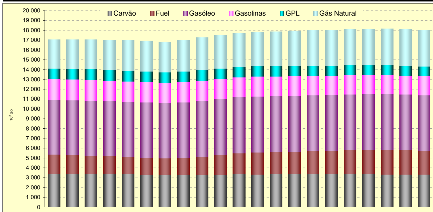
Ano Móvel - Consumo Global de Combustíveis no Mercado Interno (10 3 tep)
